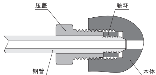
锥面螺纹接头
