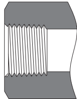
ISO 锥管阴螺纹 (FRT)
