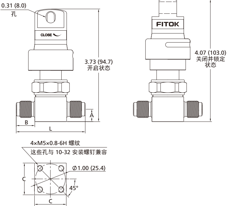
整体锁定手柄
