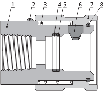
母接头
