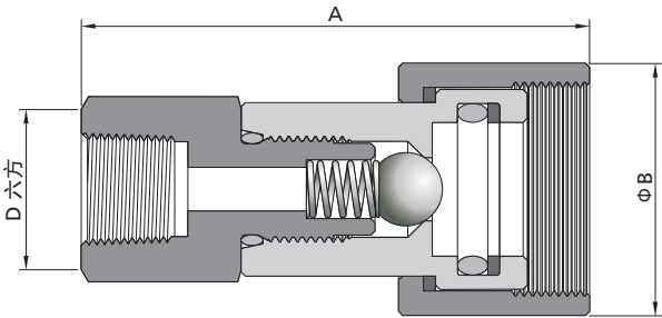
母接头
